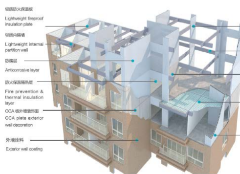
▲ 钢管混凝土束组合结构住宅建筑体系
